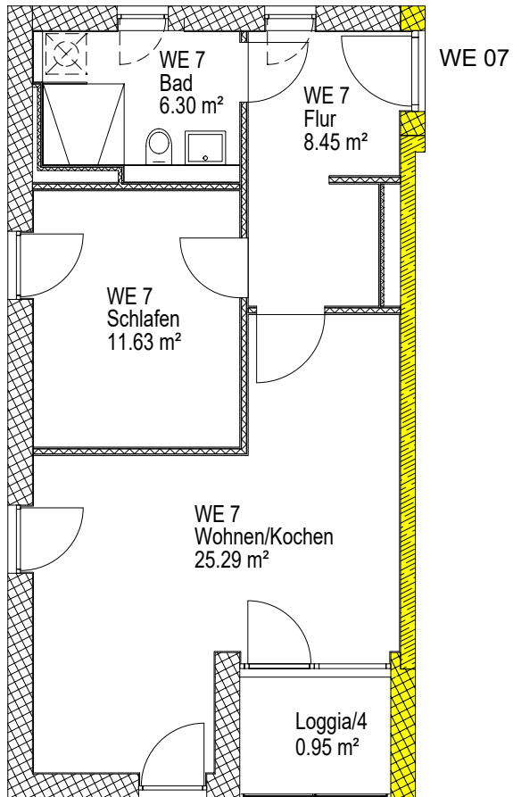
WE 07 1.OG 2-Zimmer 52.62 m 2
