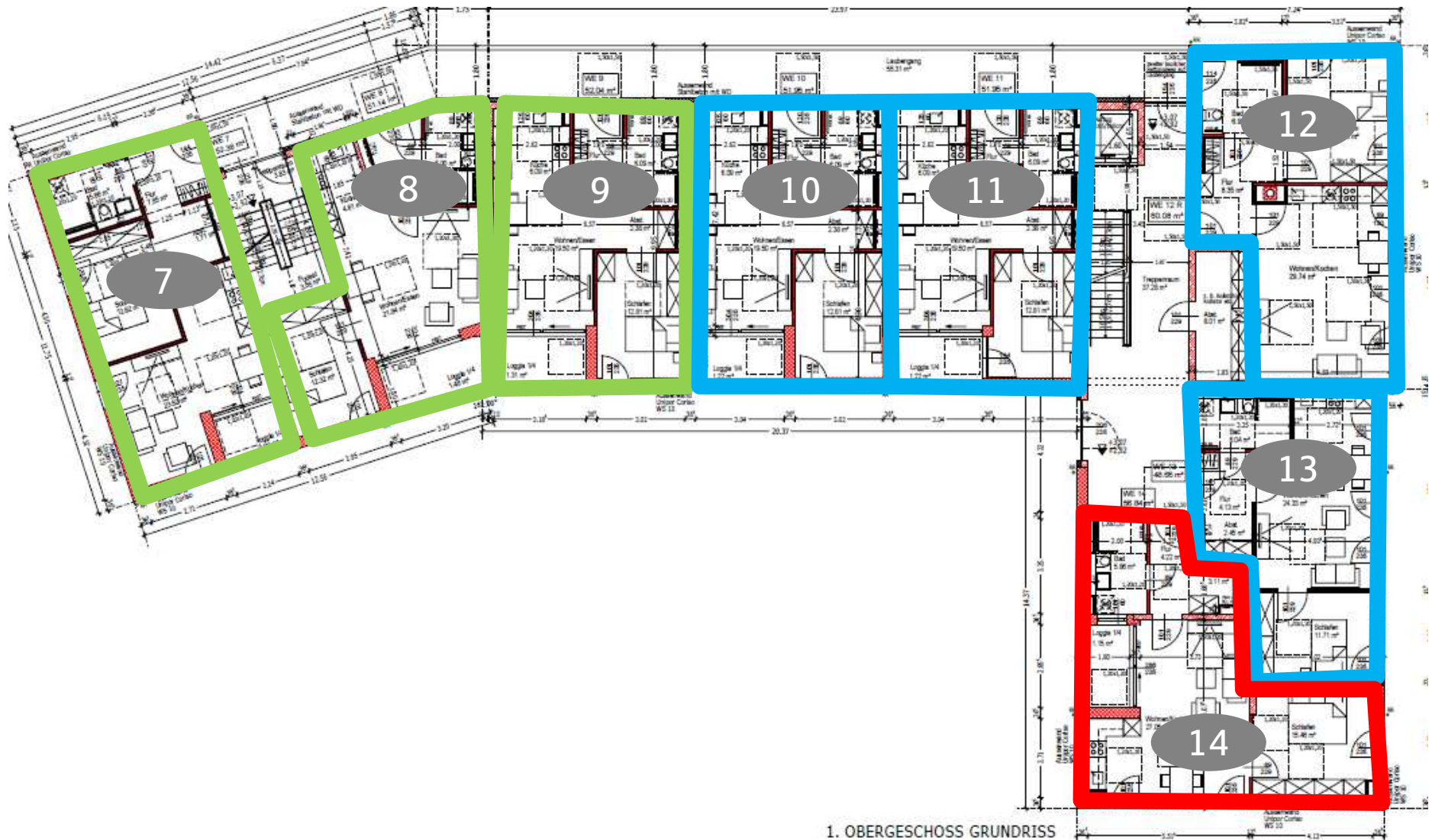
1. OBERGESCHOSS GRUNDRISS
